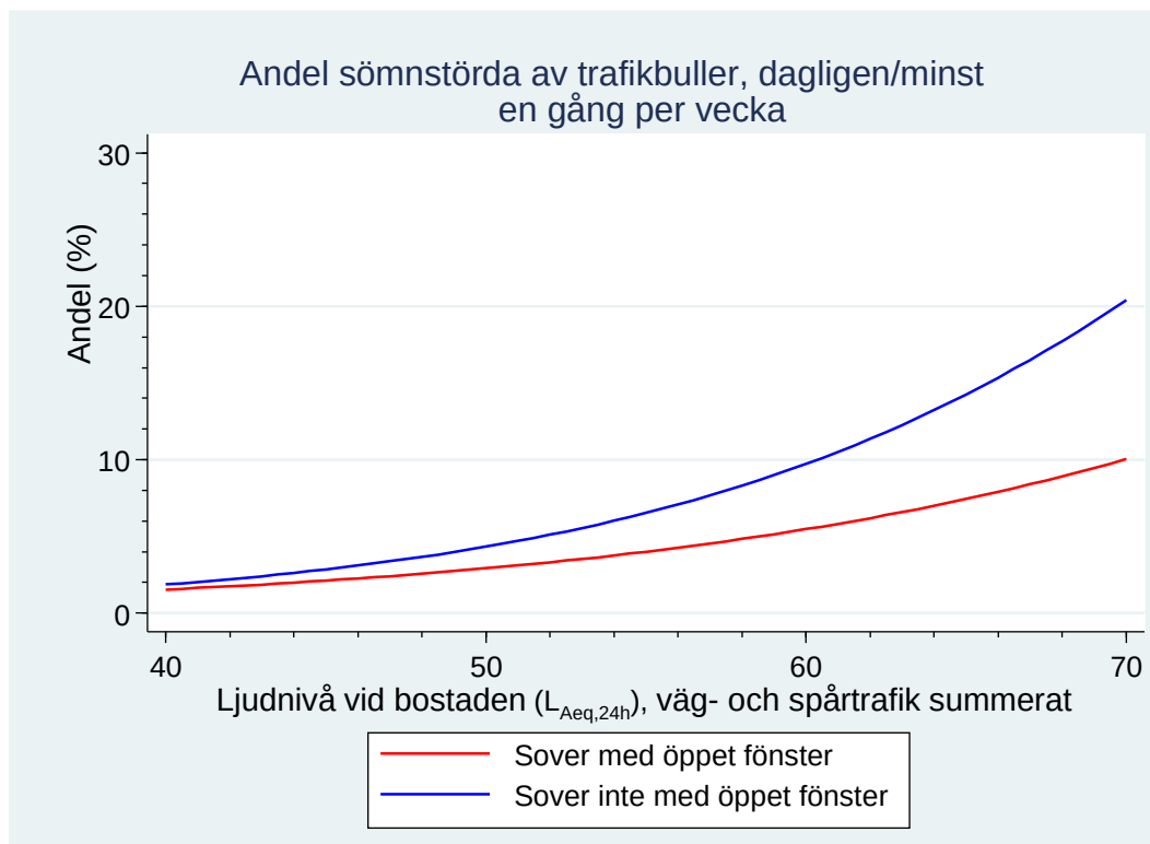
Figur 12: Exponering-responssamband mellan ljudnivå från väg- och spårtrafik utomhus vid bostaden och andel (%) i MHE 15 Stockholms län som minst en gång per vecka upplever sömnstörning till följd av trafikbuller (personer som exponeras för flygbuller \geq 40 dB FBN exkluderade), uppdelat på om man sover med öppet fönster eller ej ( p < 0,0001 ).
