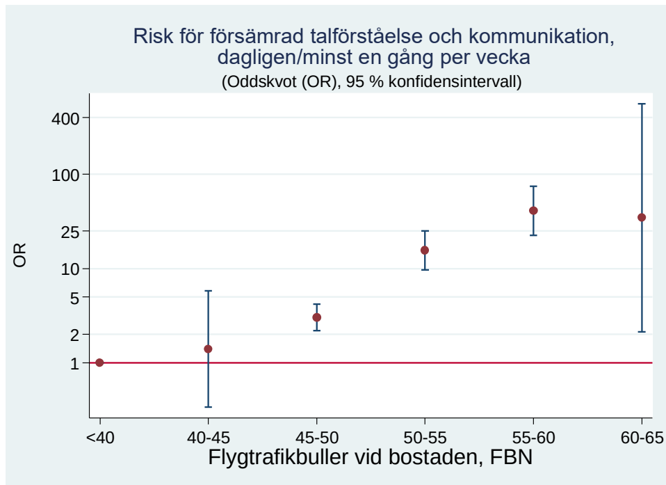
Figur 5. Risk (OR) för försämrad talförståelse och kommunikation i relation till ljudnivån utomhus vid bostaden för a) vägtrafik, b) spårtrafik och c) flygtrafik.
