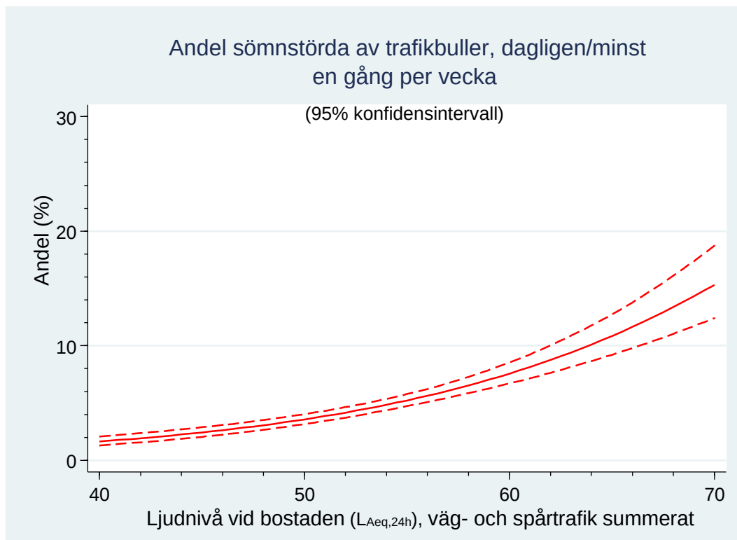
Figur 11: Exponering-responssamband mellan ljudnivå från väg- och spårtrafik utomhus vid bostaden och andel (%) i MHE 15 Stockholms län som minst en gång per vecka upplever sömnstörning till följd av trafikbuller (personer som exponeras för flygbuller \geq 40 dB FBN exkluderade).
