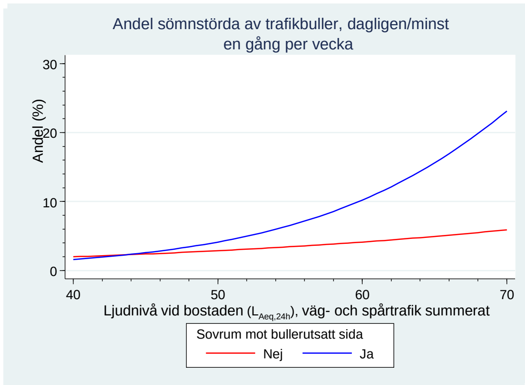
Figur 13: Exponering-responssamband mellan ljudnivå från väg- och spårtrafik utomhus vid bostaden och andel (%) i MHE 15 Stockholms län som minst en gång per vecka upplever sömnstörning till följd av trafikbuller (personer som exponeras för flygbuller \geq 40 dB FBN exkluderade), uppdelat på om sovrummet är vänt mot en bullerutsatt sida eller ej ( p < 0,0001 ).
